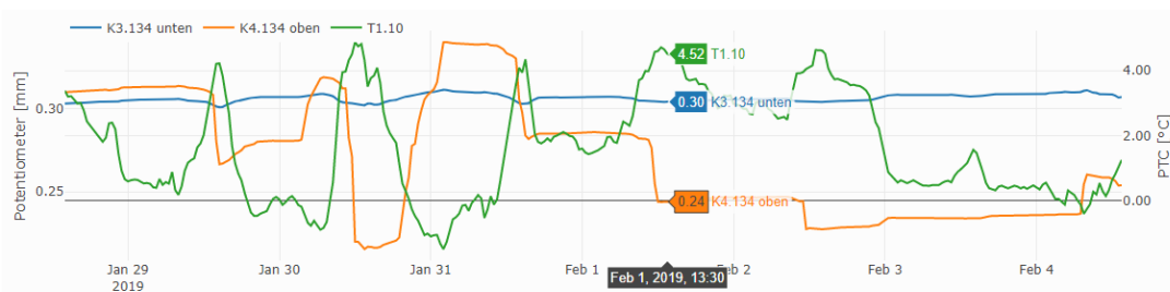
Bild 2: Verschiebungen in mm und Temperatur in °C
