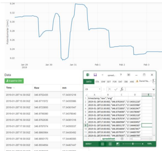
Bild 4: Wertetabelle (entweder Roh- oder technische Einheiten)
