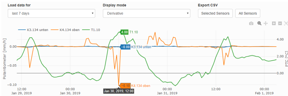
Bild 3: Verschiebungsgeschwindigkeit in mm/h und Temperatur in °C
