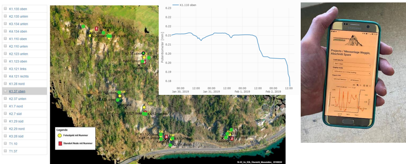
Bild 1: Mit Telejointmetern instrumentierte Felswand (Grüne Symbole der Messstellen) und Ansicht Mobile Device
